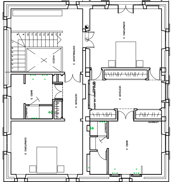
PLANTA PISO E S C. 1:150
